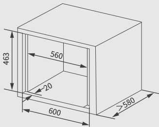
橱柜全嵌尺寸图
