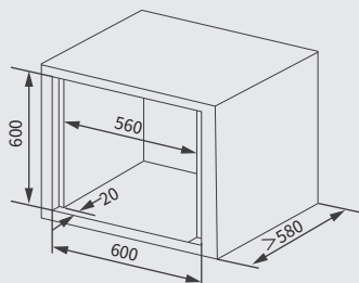
橱柜全嵌尺寸图
