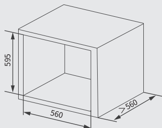
橱柜半嵌尺寸图
